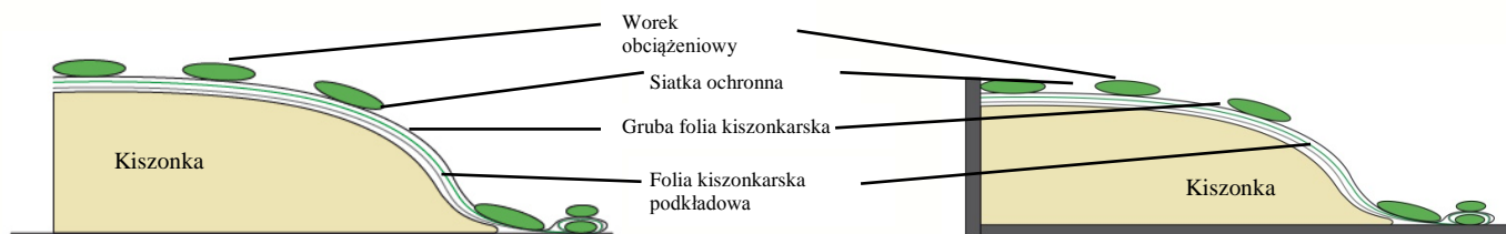
Schemat 3 : przekrój podłużny Silos pryzma / Silos korytarz
