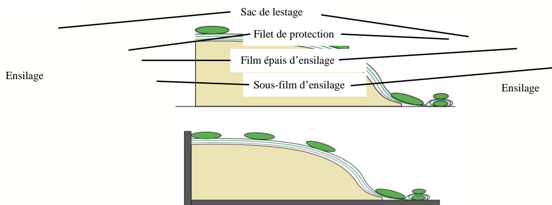
Schéma 3 : coupe longitudinale Silo taupinière / Silo couloir
