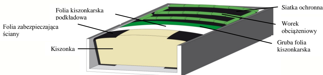
Schemat 2 : silos korytarz
