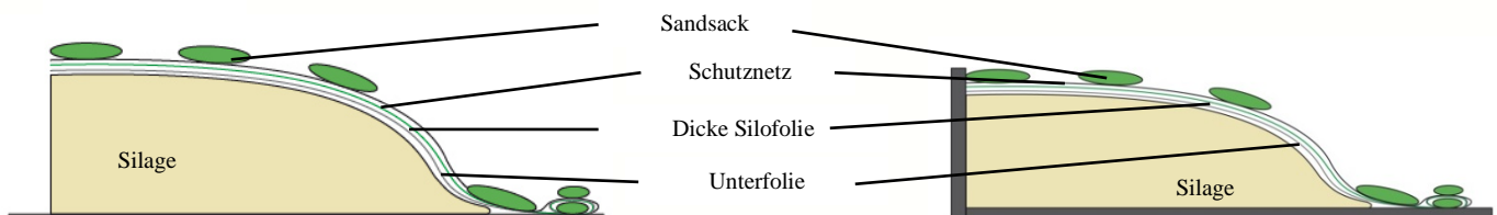
Zeichnung 3: Längsschnitt durch eine Feldmiete / ein Fahrsilo
