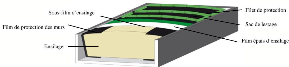
Schéma 2 : silo couloir
