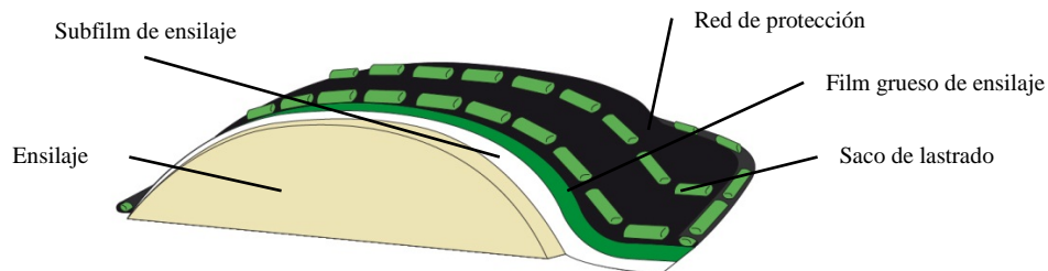
Esquema 1: Silo semienterrado
