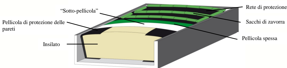
Schema 2: silo orizzontale detto "a corridoio"
