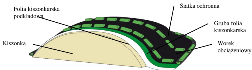
Schemat 1 : Silos pryzmowy
